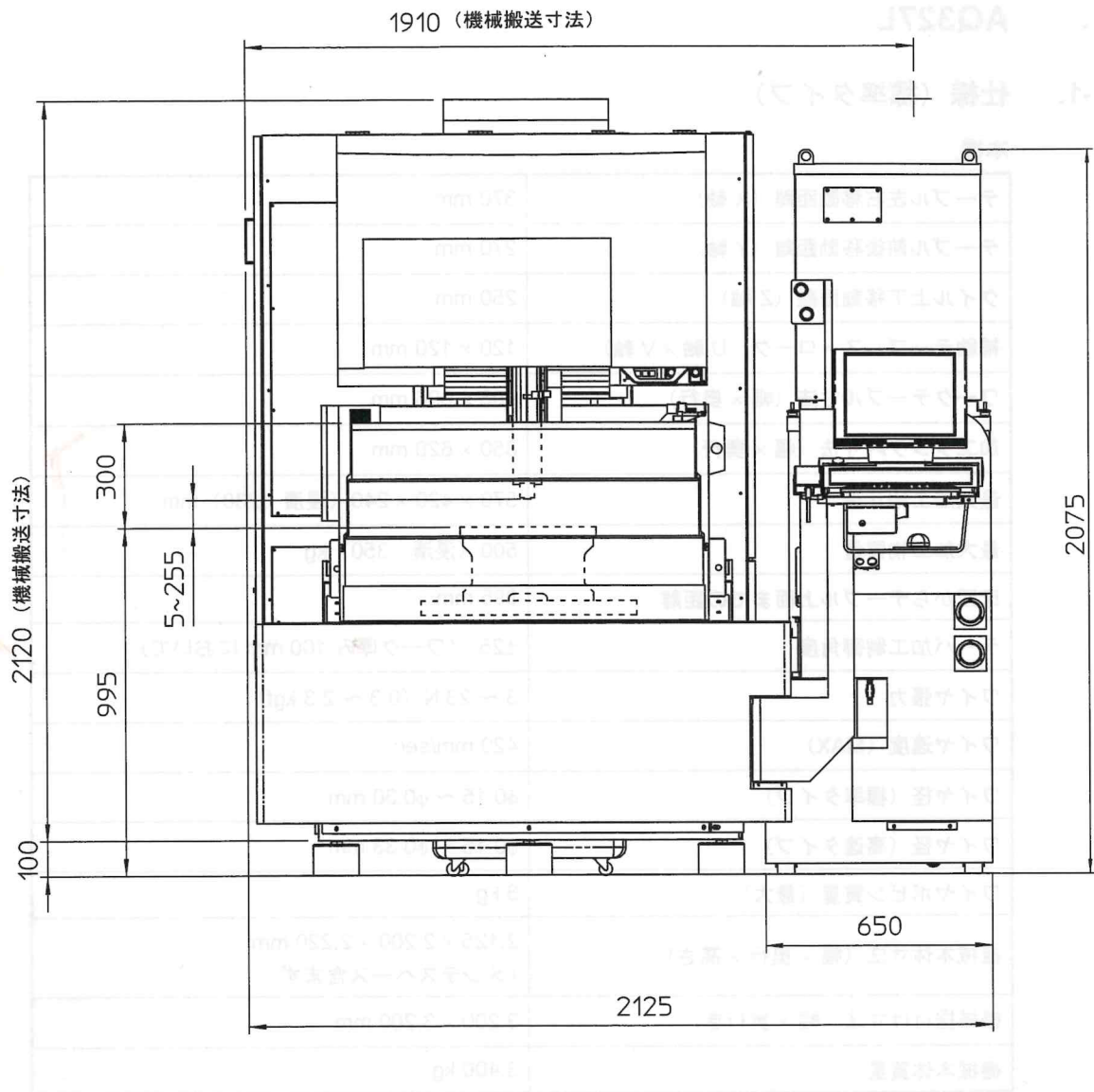
図 2-1 正面図
