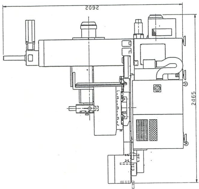
外形図
